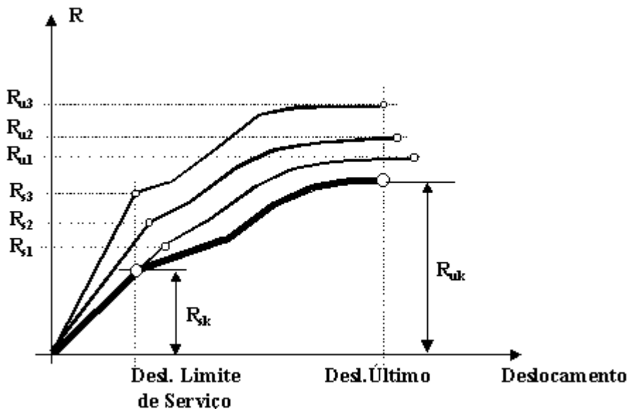
Figura B.1 – Gráfico carga x deslocamento para determinação de R_{ud} e R_{sd} por meio de ensaios
